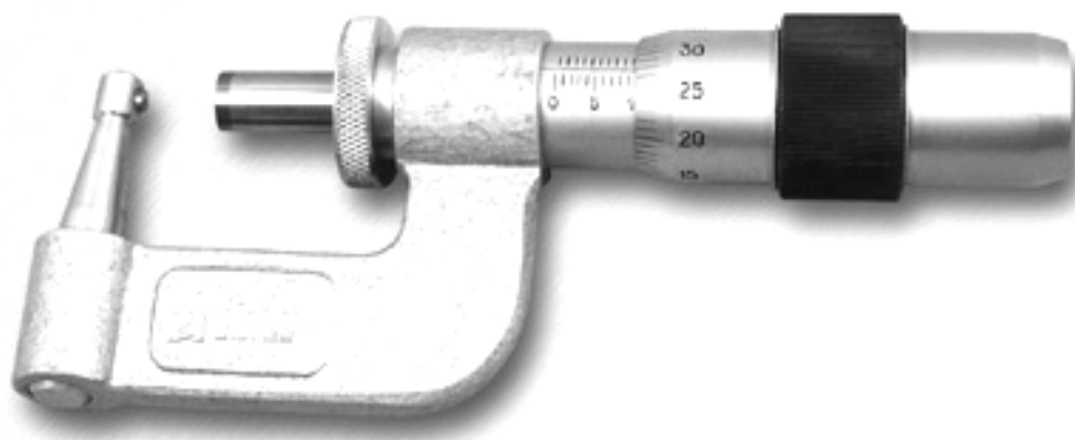
Рисунок 5 – Общий вид микрометров МГ
